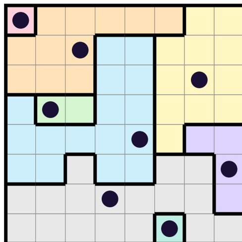
Puzzle 6 · Hard · 8×8
