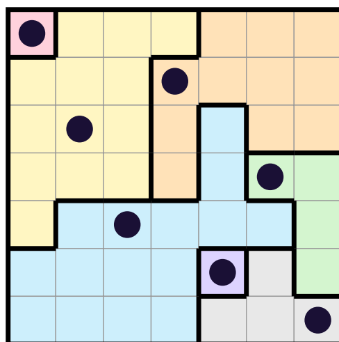
Puzzle 4 · Medium · 7×7
