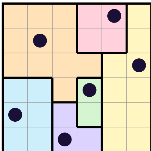
Puzzle 1 · Easy · 6×6
