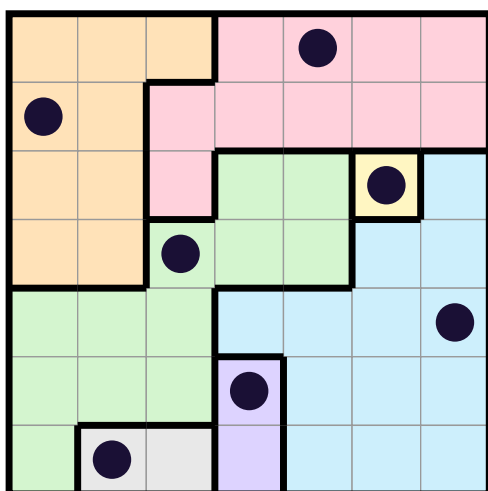
Puzzle 3 · Medium · 7×7
