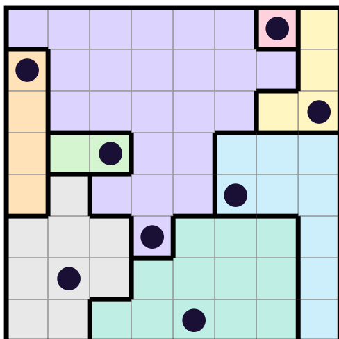
Puzzle 5 · Hard · 8×8
