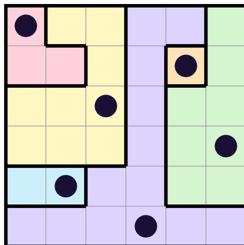
Puzzle 2 · Easy · 6×6
